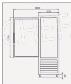
VISTA LATERALE Side view / Seitenansicht / Vue latérale
